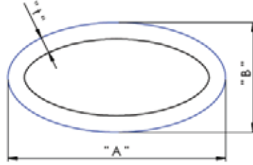
Elips Profil
