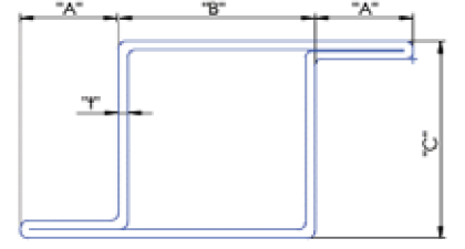
Z-Profil
